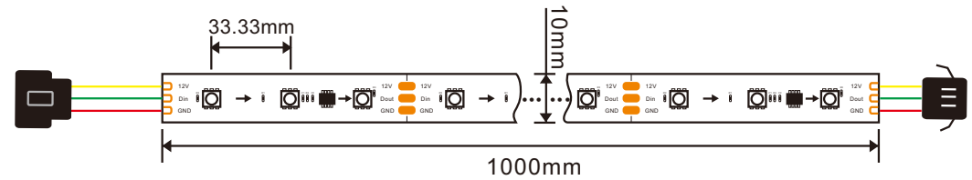
60LEDS
